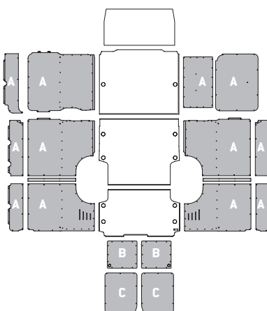
Modelo - Model L5 H2 / XLH2
