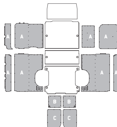
Modelo - Model L4 H2 / LH2
