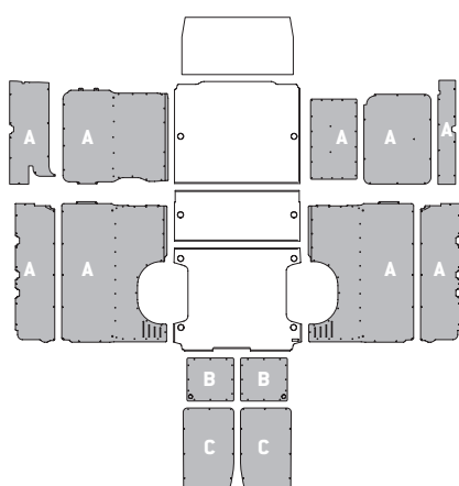
Modelo - Model L4 H3 / LH3
