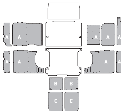
Modelo - Model L1 H2 / CH2
